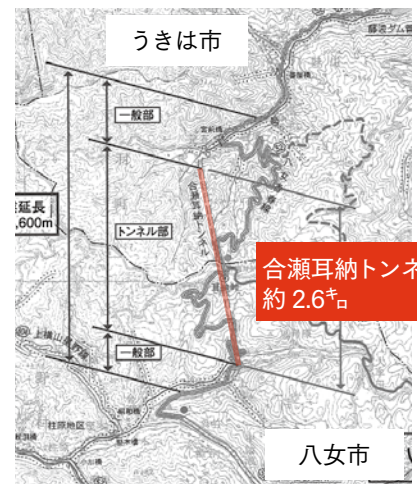
▼合瀬耳納トンネルの位置図
