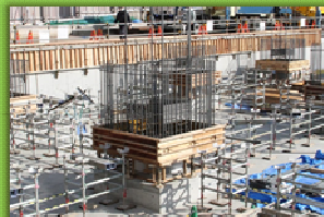
免震装置上基礎
