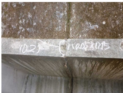
熊の内3号ロックシェッド (主梁の剥離・鉄筋露出：Ⅱ)
