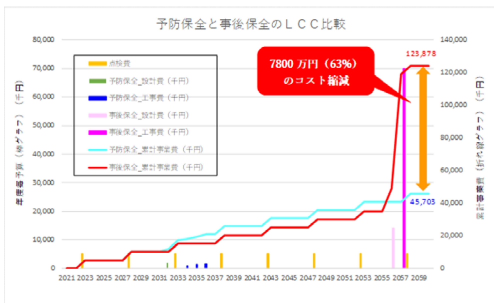
予防保全と事後保全のライフサイクルコスト比較（シェッド）
