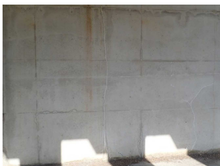
熊の内ロックシェッド (山側受台のひびわれ：Ⅱ)
